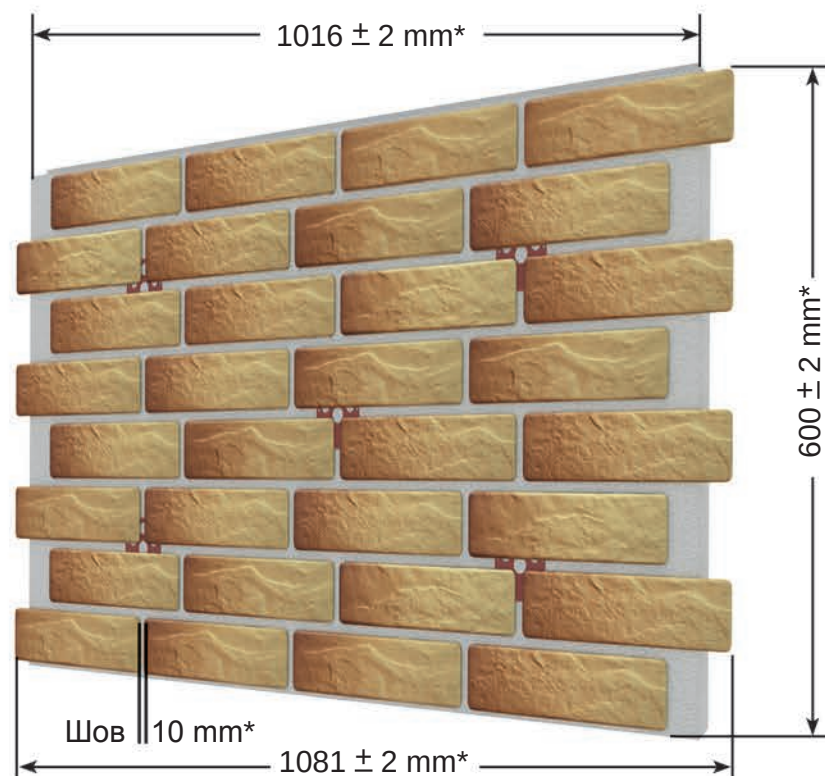
Прямий елемент 1/4
