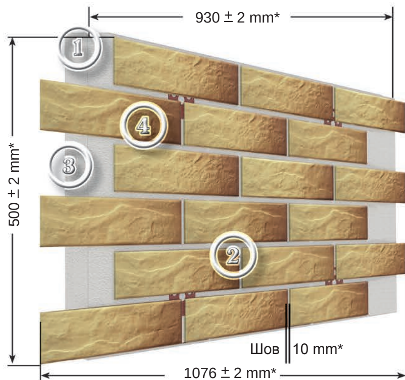
Прямий елемент 1/2
