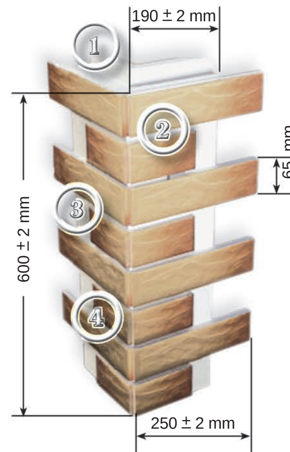
Кутовий елемент 1/2
