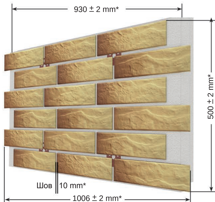
Прямий елемент 1/4
